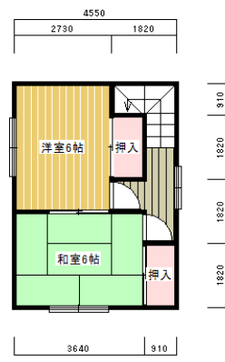
2階平面図
