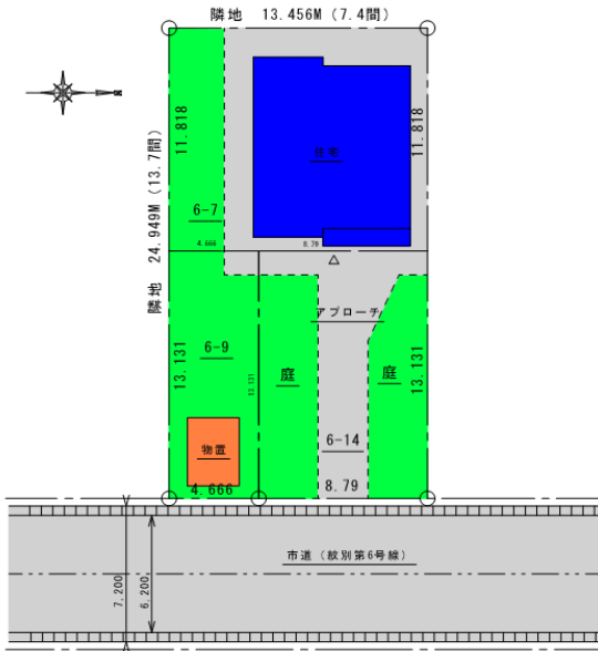
敷地図
