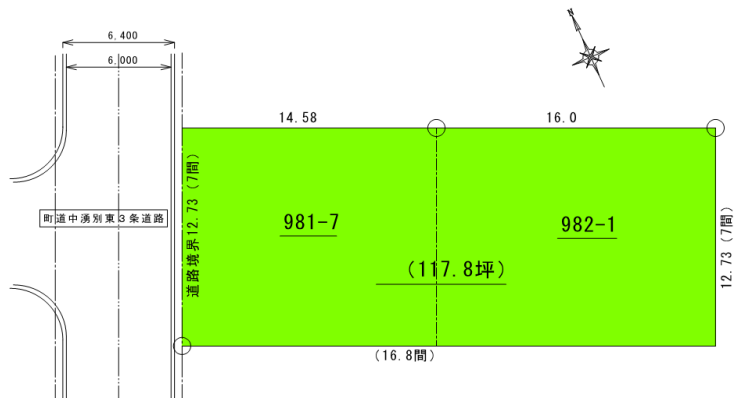
敷地図
