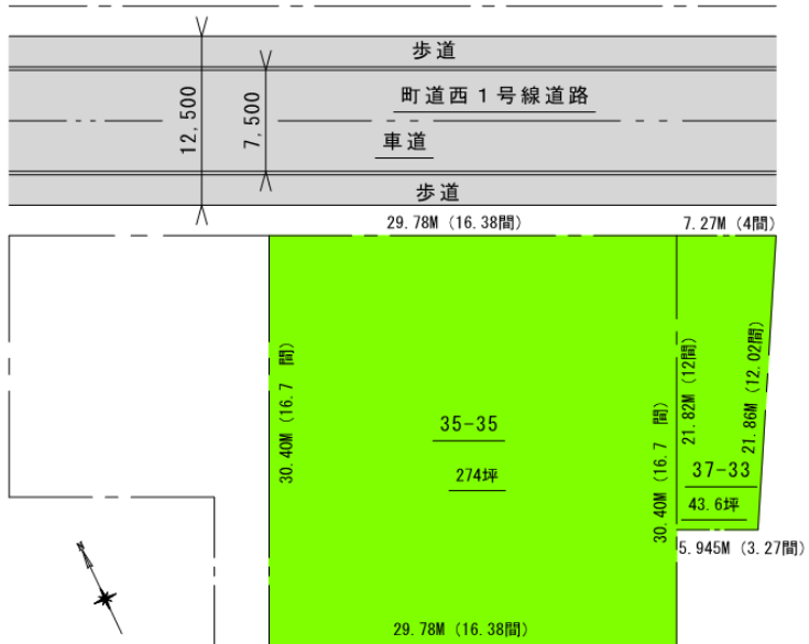
付近見取図
