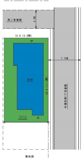
敷地図
