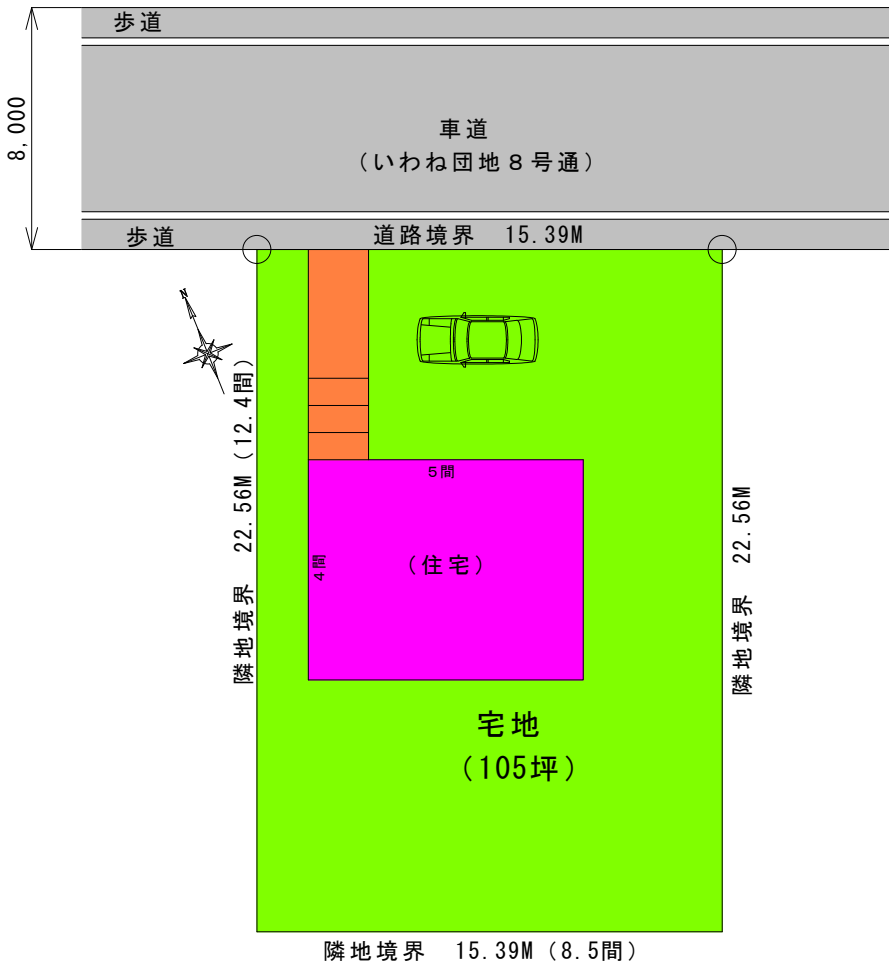
配置例
